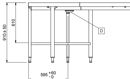
Oldalnézet
