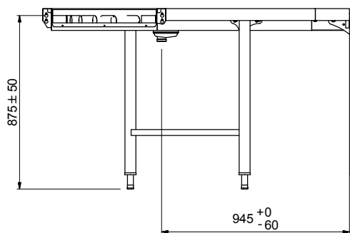
Oldalnézet
